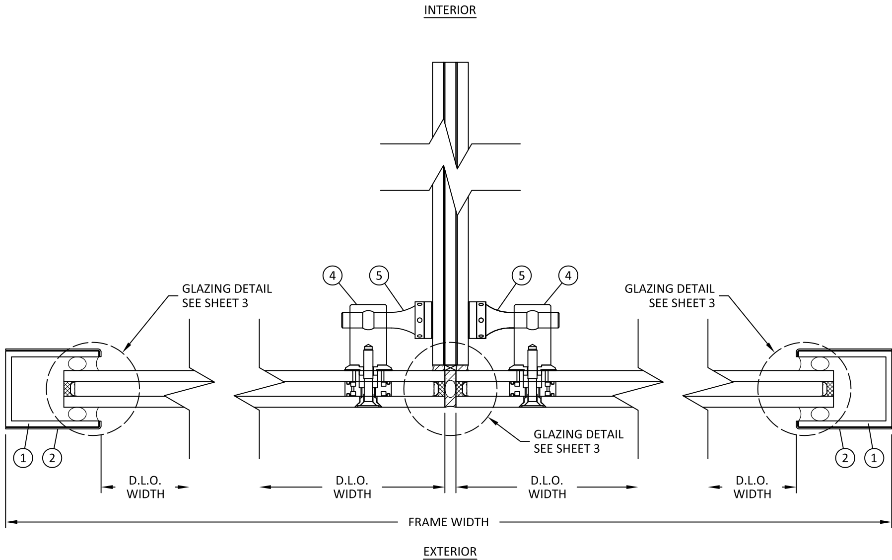
E 5 HORIZONTAL SECTION JAMB
